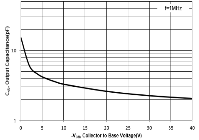
Fig. 6 Output Capacitance
