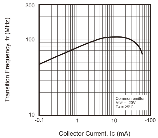
Fig.6 - f_T — I_C
