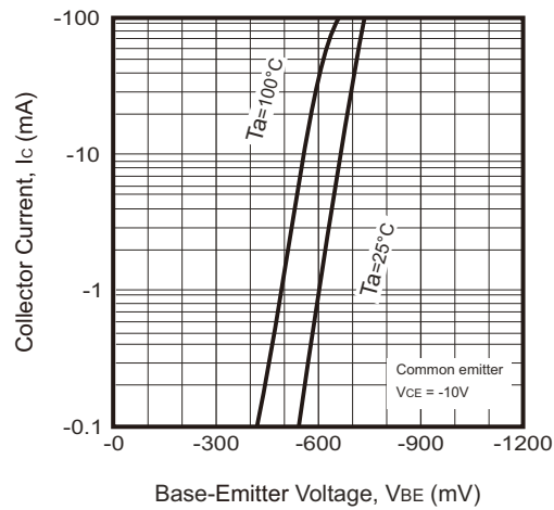
Fig.5 - I_C — V_{BE}
