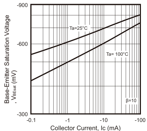
Fig.4 - V_{BEsat} - I_C
