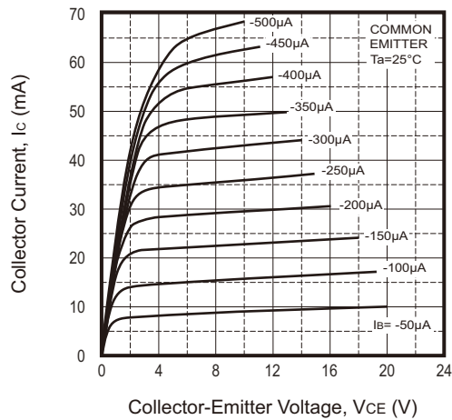
Fig.1 - I_C - V_{CE}
