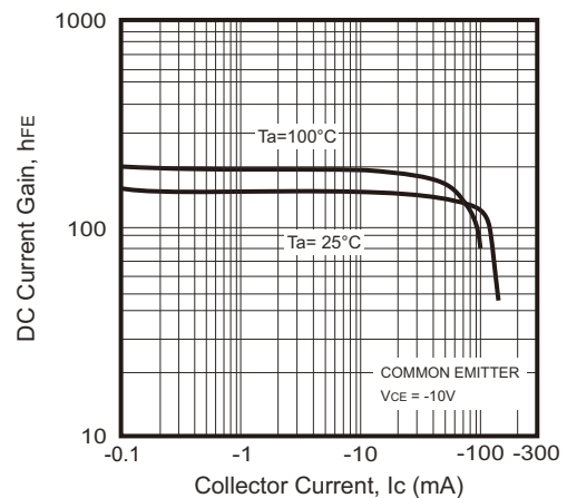
Fig.2 - h_{FE} - I_C
