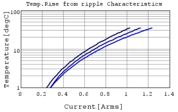
GRT1555C1H470JA02 Temp.rise 500MHz
