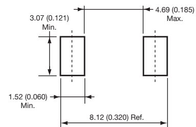
DO-214AB (SMC)
